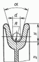
Н: 1,33—1,75 d . \alpha — угол развала желоба шкива 30°—50°.
