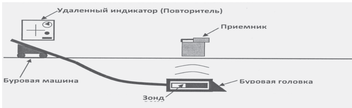
Рисунок В.2 – Схема действия электромагнитной системы подземной локации
