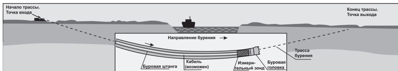
Рисунок 8.3 – Направленное бурение пилотной скважины
