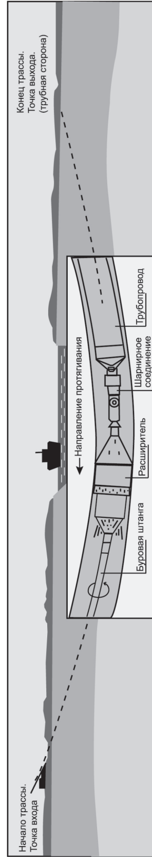
Рисунок 8.6— Сборка буровой колонны для протягивания трубопровода
