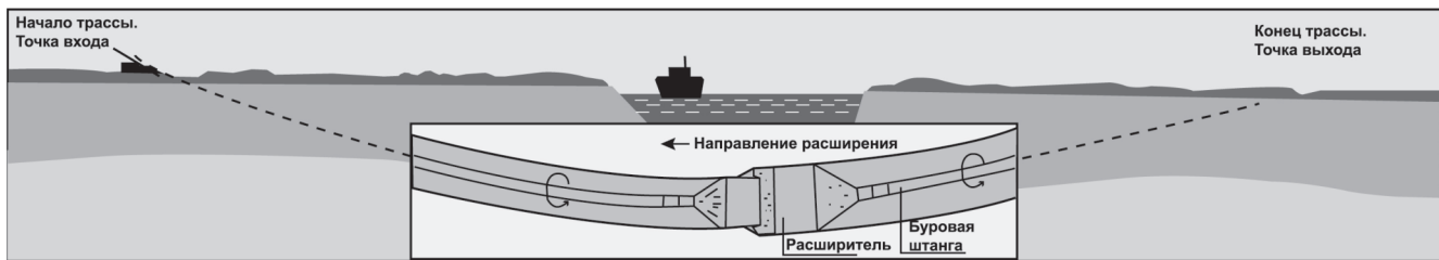
Рисунок 8.4 – Расширение скважины
