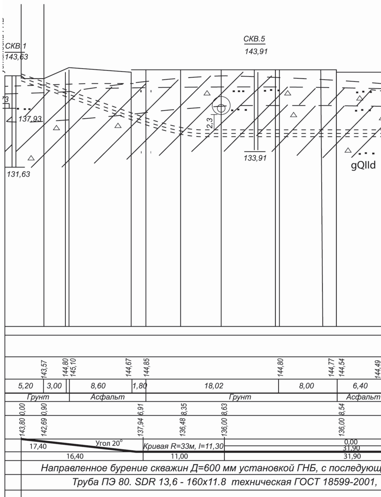
7.1 – Пример построения продольного профиля
