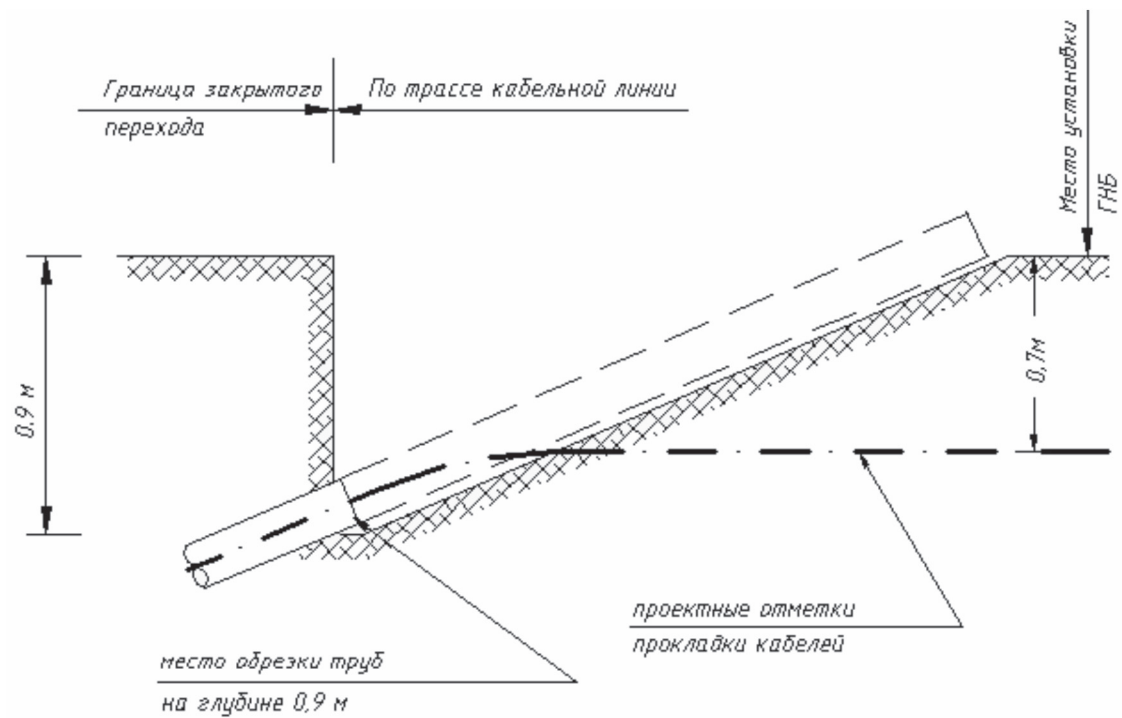
Рисунок 7.5 – Варианты шурфов для вывода кабелей из перехода
